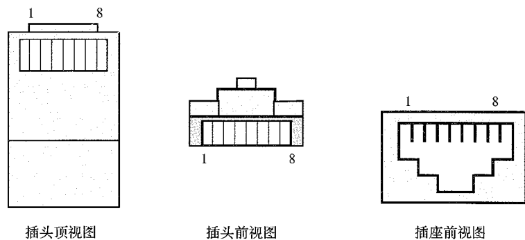
图 8.2.5 信息插座插头接线
