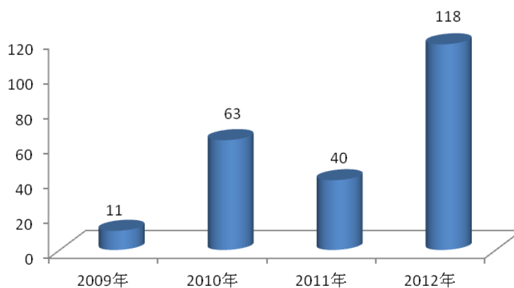
图G.3 地闪频数年分布图
